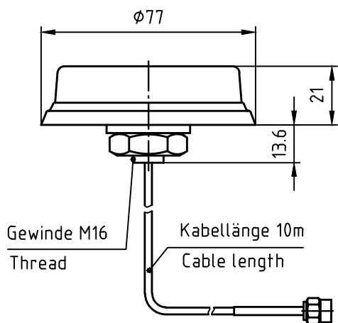
Antenna GSM 10m Teile-Nr./Part No. P8000008358
